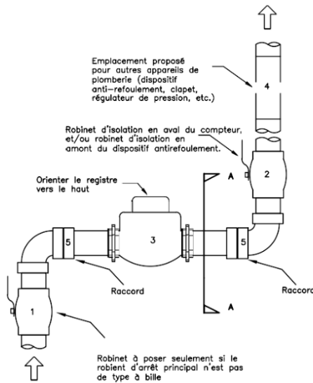
VUE DE FACE (Aucune échelle)
