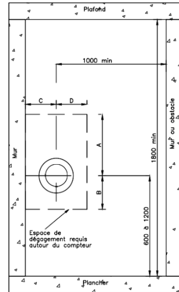
COUPE A-A (Aucune échelle) en mm
