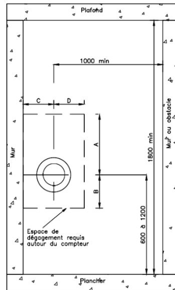
COUPE A-A (Aucune échelle) en mm
